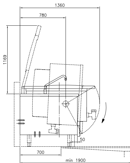
Zij aanzicht
