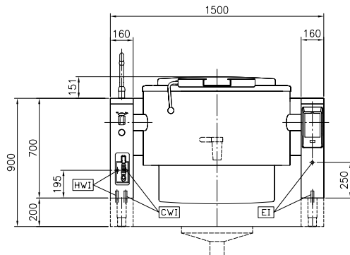
Zij aanzicht
